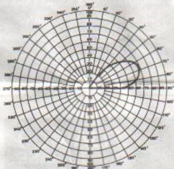
Diagrama de radiación en el plano vertical sobre tierra. Radiation pattern in the vertical plane on earth. Diagramme de rayonnement en plan vertical au sol.
