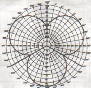
Diagrama de radiación en el plano horizontal Horizontal radiation pattern Diagramme de rayonnement dans le plan horizontal
